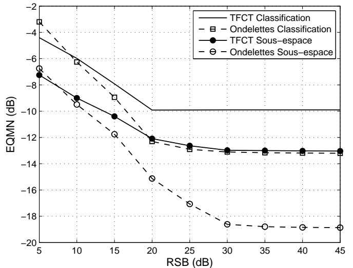
FIG. 2 – Performances de l'algorithme de séparation de 4 sources audio pour 3 capteurs : les courbes représentent la valeur moyenne de l'erreur quadratique de l'estimation des signaux sources en fonction du rapport signal à bruit.
