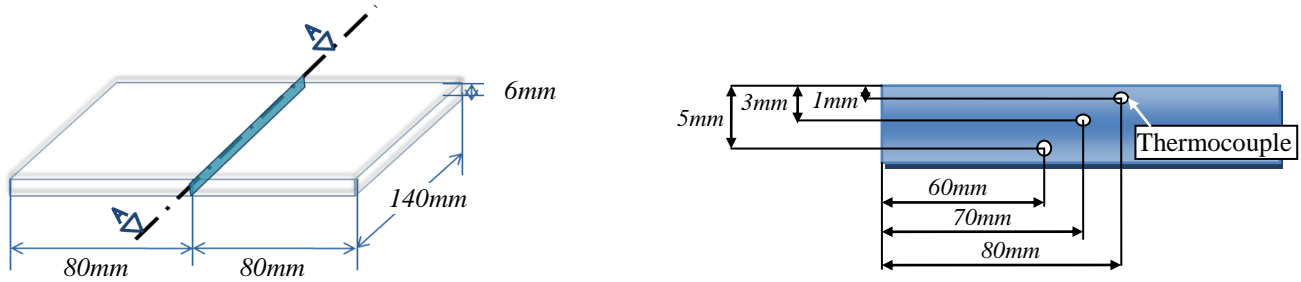
Figure 11 - Positions des thermocouples selon l'épaisseur du composite
