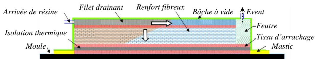
Figure 2 - Présentation schématique du LRI
