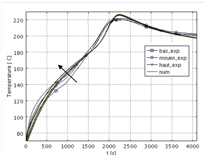
Figure 12 - Variation de la température en fonction du temps en trois points dans l'épaisseur
