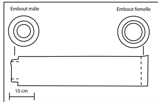
St007004207, tuyan en terre cuite, musée Rolin (L.B.)
