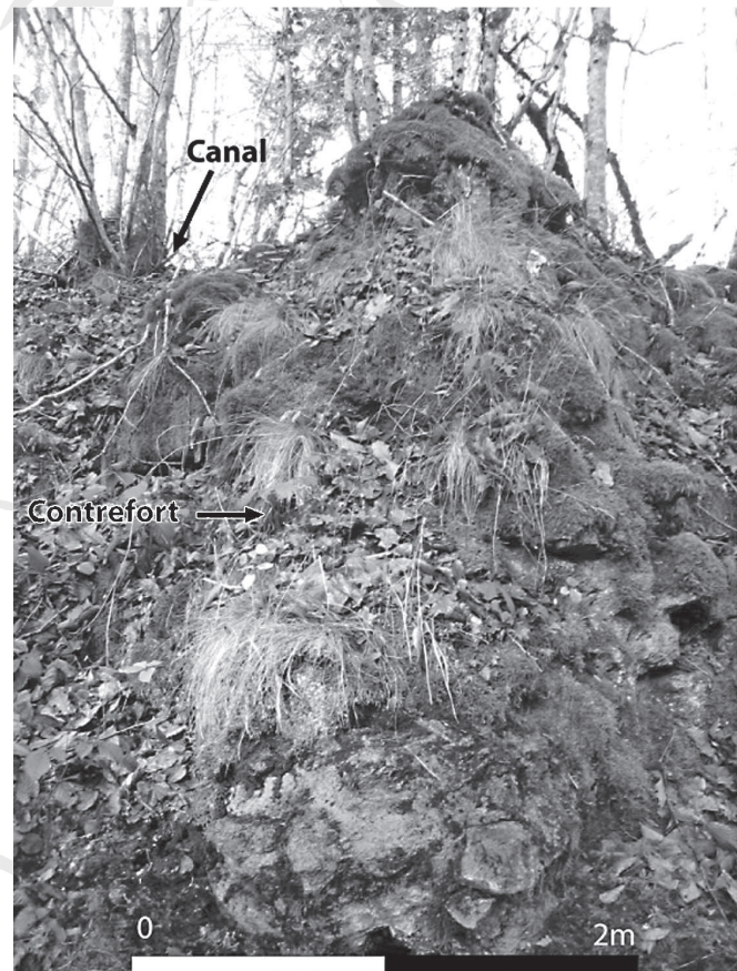
Fig. 5. Contrefort St 029 installé dans la pente en contrebas du canal (cl. L. Borau).
