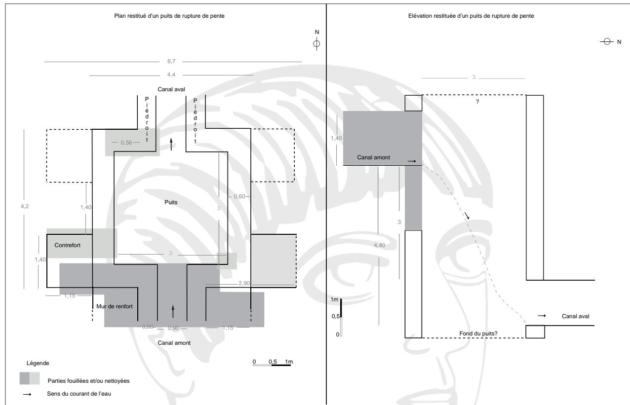
Fig. 6. Restitution d'un puits de rupture de pente, vu en plan et en coupe (DAO L. Borau).
