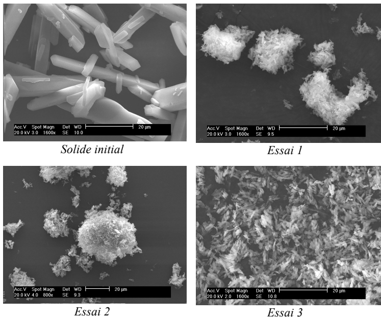
Figure 4. Images MEB du solide initial et recristallisé (Essais 1, 2 et 3).
