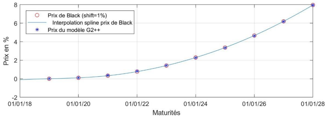
Figure 14 : qualité de reproduction des prix de caps par le modèle de G2++ (G2, décalage=1%)
