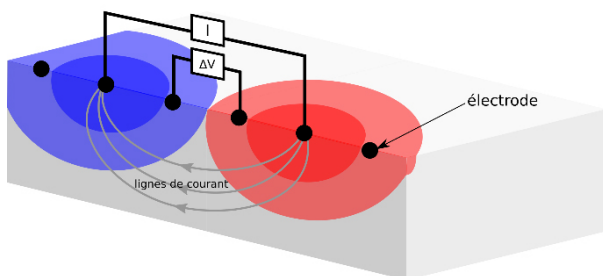
a) Tomographie de Résistivité Électrique (TRE)
