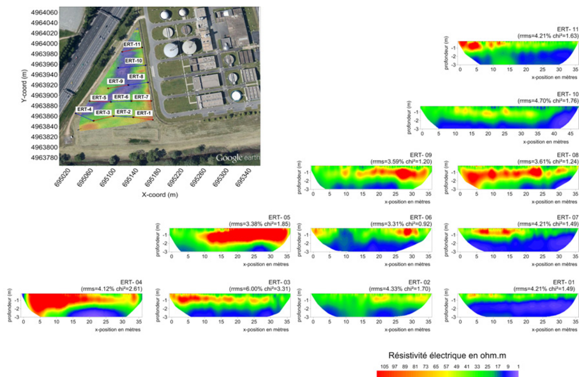
Figure 8 : Profils de TRE obtenus sur le site de Bègles. Le plan en haut à gauche reprend les résultats de conductivité électromagnétique et situe les différents profils de TRE
