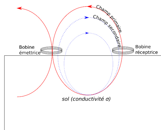
b) Conductimétrie électromagnétique
