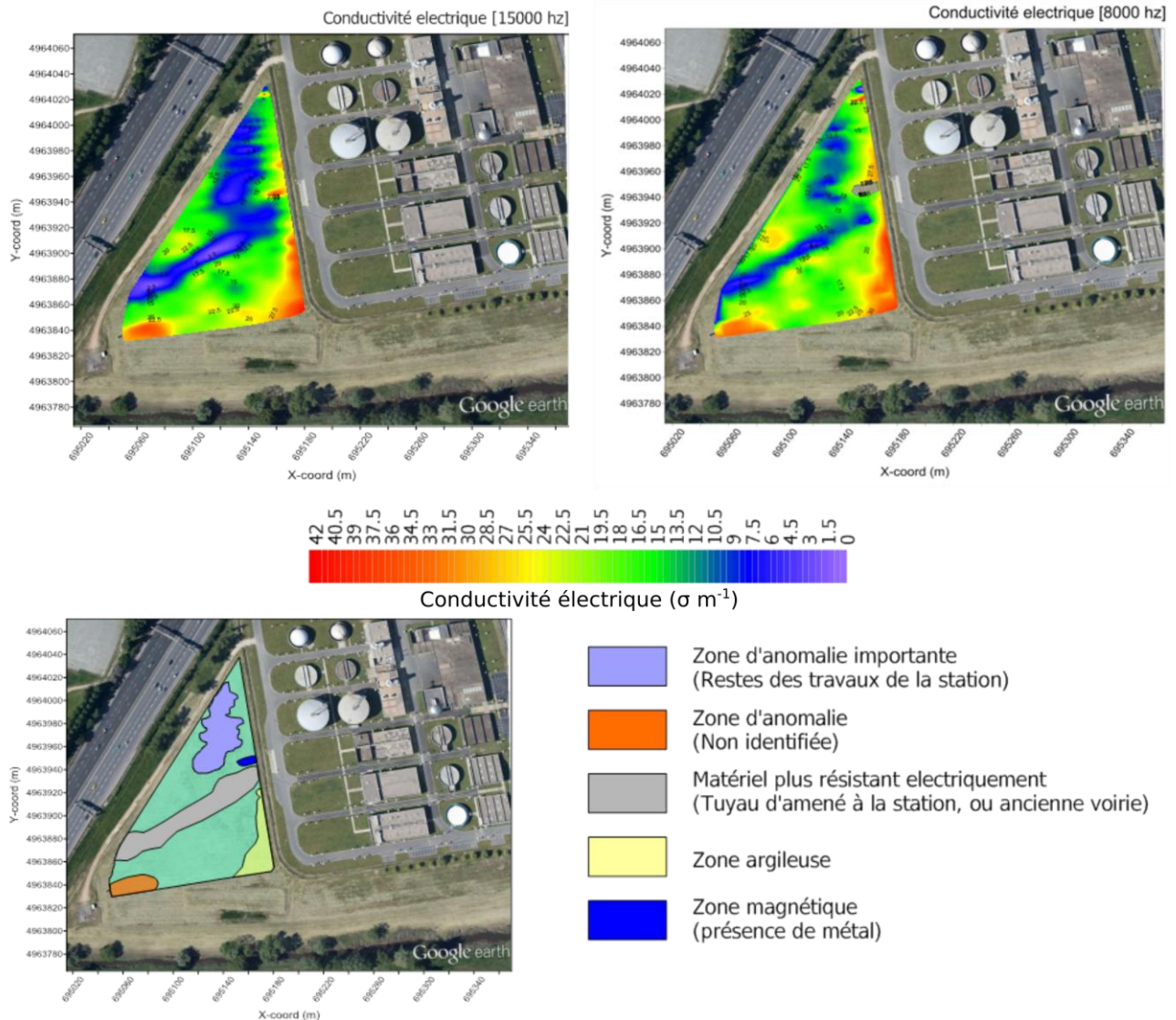
Figure 7. Résultats du conductimètre électromagnétique à 8000 Hz et 15000 Hz et définition du Plan 1
