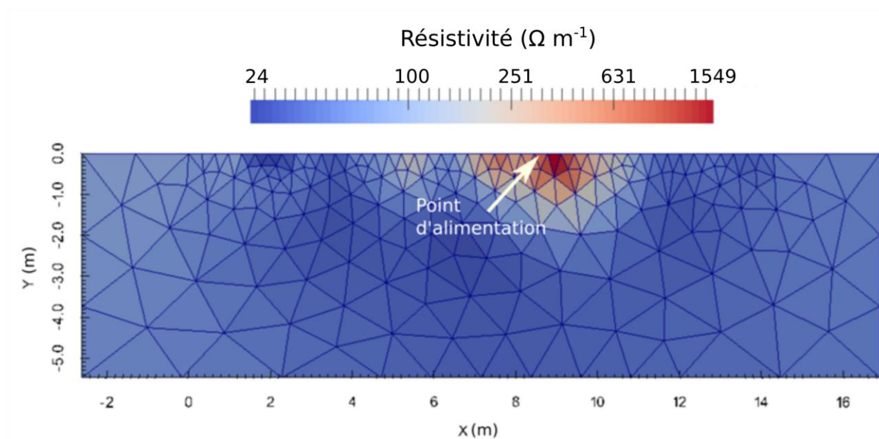
Figure 4: Coupe obtenue par TRE mettant en évidence une anomalie au niveau du point d'alimentation de l'aire d'infiltration
