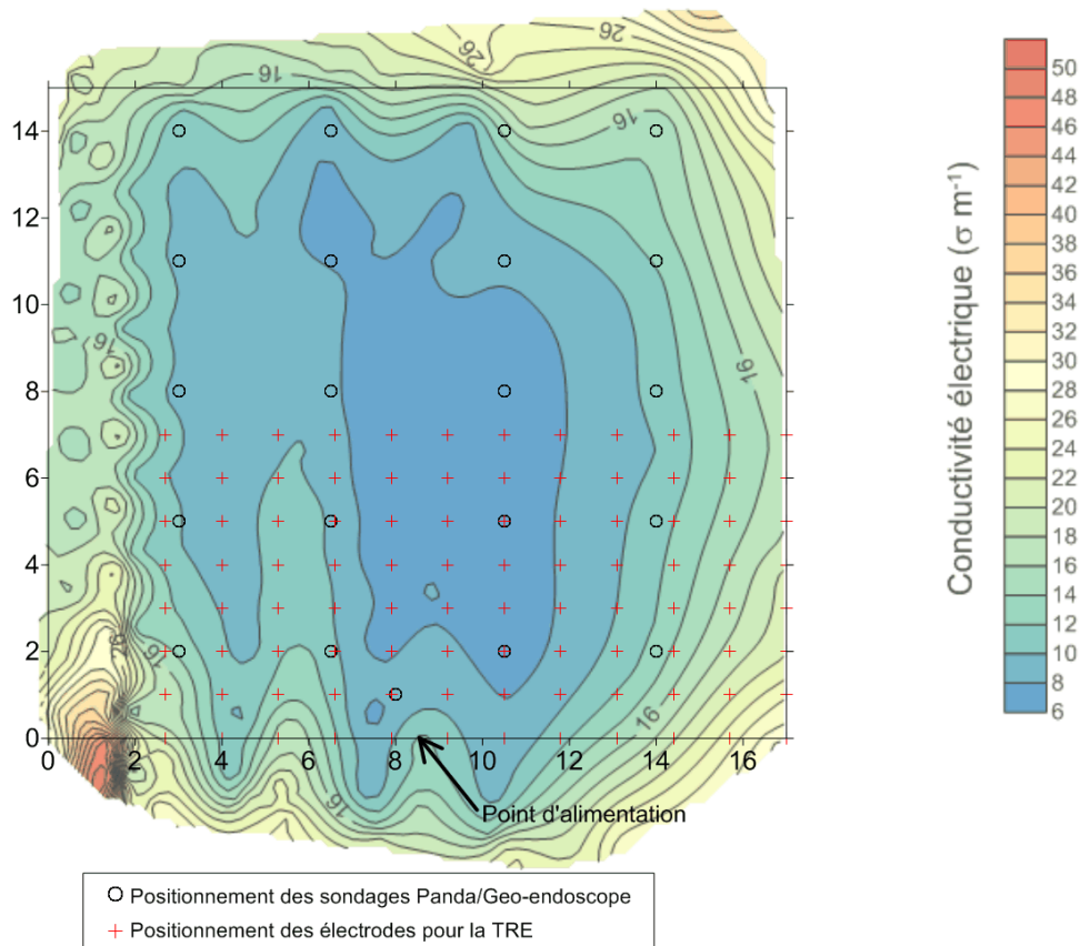
Figure 3. Résultats de la mesure de la conductivité électrique et positionnement des électrodes de la tomographie de résistivité électrique ainsi que des sondages de pénétrométrie et de géo-endoscopie
