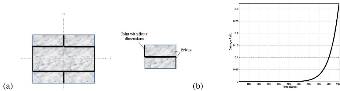
FIGURE 1 – Cellule de maçonnerie périodique avec des joints de dimensions finies constitués de mortier viscoélastique micro-fissuré et son quart (a) considéré pour la modélisation avec une évolution temporelle non linéaire de l’endommagement accumulé (14) [28] (b) dans les joints.
