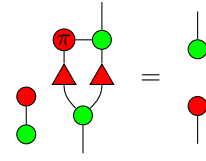
Lemma 25.
