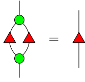
Lemma 22.
