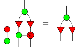
Lemma 24.
