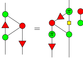
Lemma 24.
