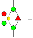
Lemma 22.
