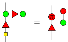
Lemma 20.
