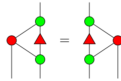
Lemma 17.
