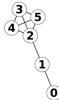
Fig. 3. The lollipop L_6 .
