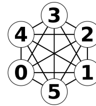
Fig. 2. The clique K_6 .
