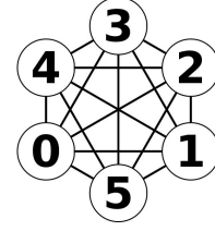
Fig. 2. The clique K_6 .
