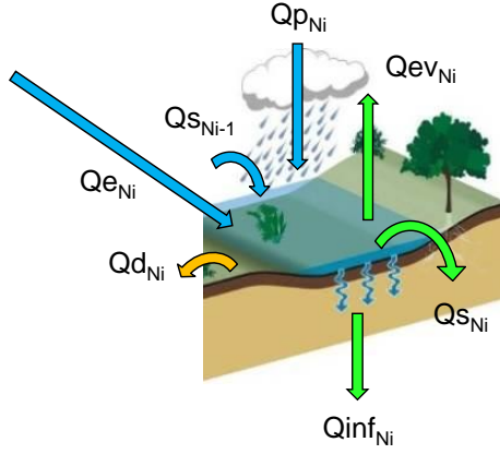
Figure 3. Schéma de fonctionnement d'une noue dans le scénario S2. (complété à partir de http://guidebatimentdurable.bruxellesenvironnement.be ).
