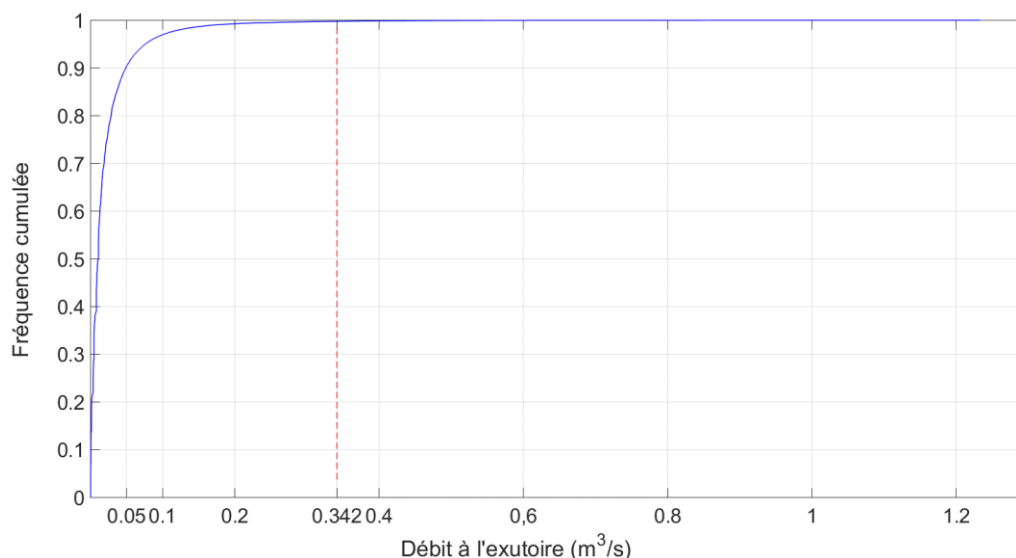
Figure 11. Distribution cumulée des débits à l'exutoire dans le scénario S1.
