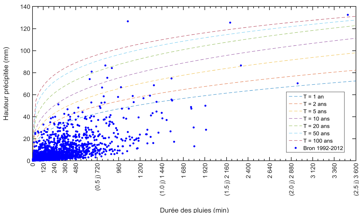
Figure 8. Diagramme durée – hauteur des événements pluvieux de la chronique 1992-2012 à Bron. Les courbes HDF correspondent aux données expérimentales du Grand Lyon.
