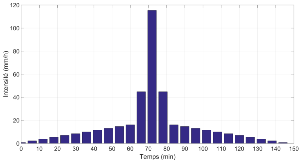
Figure 6. Pluie de projet double triangle utilisée dans le scénario S1, discrétisée au pas de temps de 6 minutes (source SEDic).
