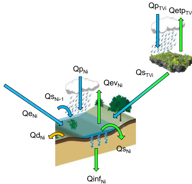
Figure 5. Schéma de fonctionnement d'une noue et d'une toiture végétalisée dans le scénario S3 (complété à partir de http://guidebatimentdurable.bruxellesenvironnement.be et de http://www.vegetalid.us ).
