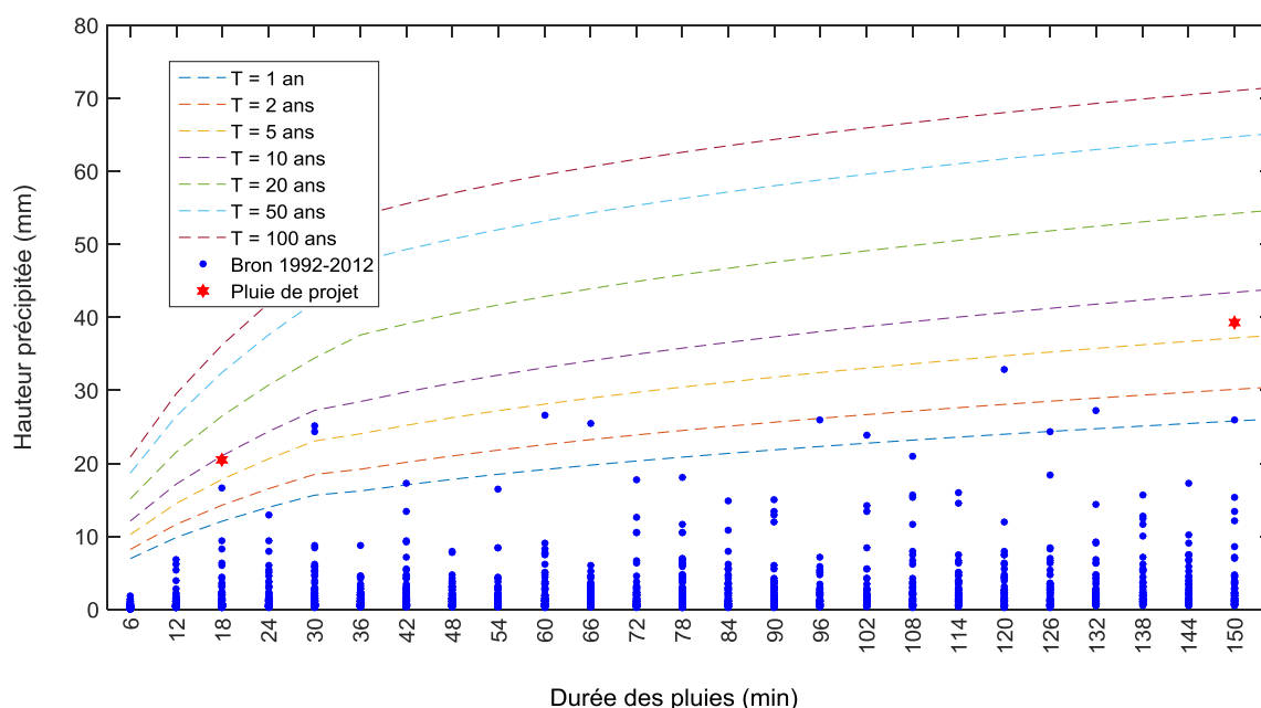
Figure 9. Diagramme durée – hauteur des événements pluvieux de la chronique 1992-2012 à Bron : zoom de la Figure 8 pour les pluies de durée de 6 à 150 minutes. Ajout de la pluie de projet (période intense sur 18 min et durée totale de 2h30 = 150 min).
