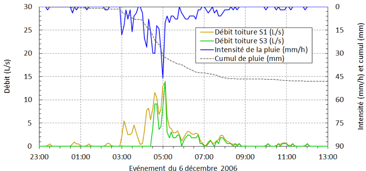
Figure 12. Débit en sortie de toiture du sous-bassin versant 1, événement du 6 décembre 2006, scénarios 1 et 3.
