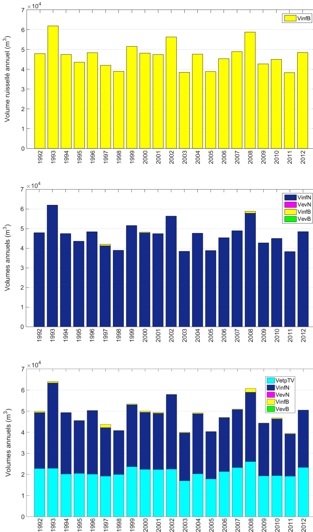
Figure 10. Bilans hydrologiques annuels pour les trois scénarios S1 à S3 du haut vers le bas.
