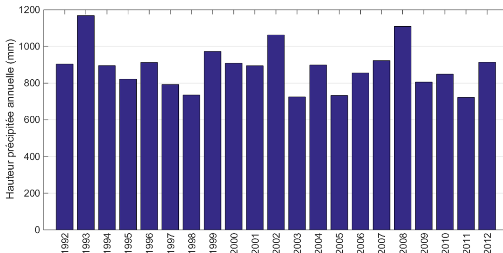
Figure 7. Pluviométrie annuelle sur la période 1992-2012.
