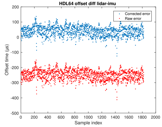
(b) HDL64e
