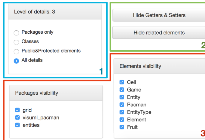
Fig. 5: VisUML Filters
