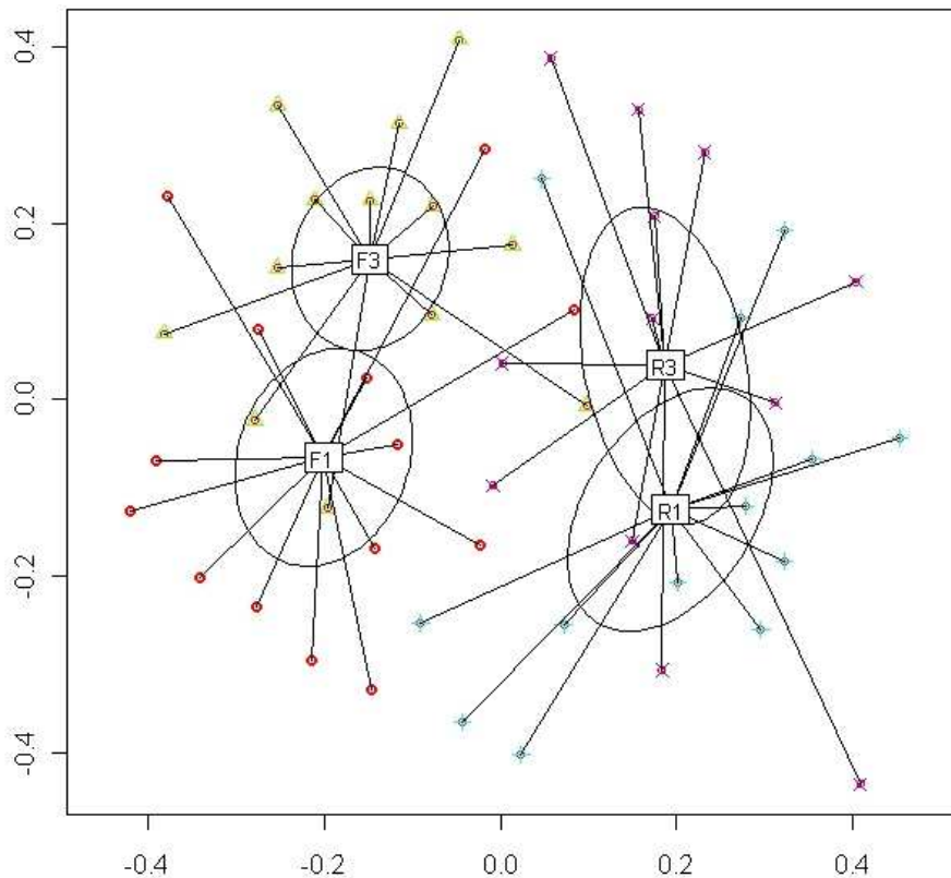
Figure 2 : Analyse multivariée (positionnement non métrique) de la composition des communautés de coléoptères saproxyliques en fonction de l'ancienneté de l'état boisé et du caractère feuillu ou résineux des peuplements, dans 52 sites en forêt d'Orléans. Même signification des libellés qu'à la figure 1. L'axe 1 (horizontal) sépare les forêts feuillues et résineuses, et l'axe 2 sépare les forêts anciennes et récentes.
