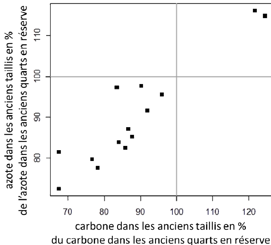
Figure 3 : Comparaison des teneurs en azote (verticalement) et carbone (horizontalement) entre les anciens taillis et anciens quarts en réserve dans 14 couples de sites du Plateau lorrain. On observe une forte baisse du taux de matière organique de l'horizon supérieur du sol dans la plupart des systèmes anciennement exploités en taillis.
