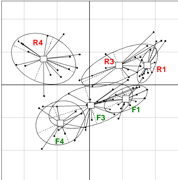
Figure 1 : Analyse canonique des correspondances de la composition floristique de 80 relevés floristiques en forêt d'Orléans (98 espèces) en fonction des 6 modalités du plan d'échantillonnage. F : feuillus ; R : résineux ; 1 : forêt déjà boisée en 1840 ; 3 : forêt boisée entre 1840 et 1949 ; 4 : forêt boisée après 1949. La modalité est placée au barycentre des relevés qui le composent. Le premier axe (horizontalement), qui explique 43% de l'inertie, sépare les relevés en fonction de l'ancienneté de l'état boisé. Le second explique 21% de l'inertie et distingue les peuplements feuillus et résineux.
