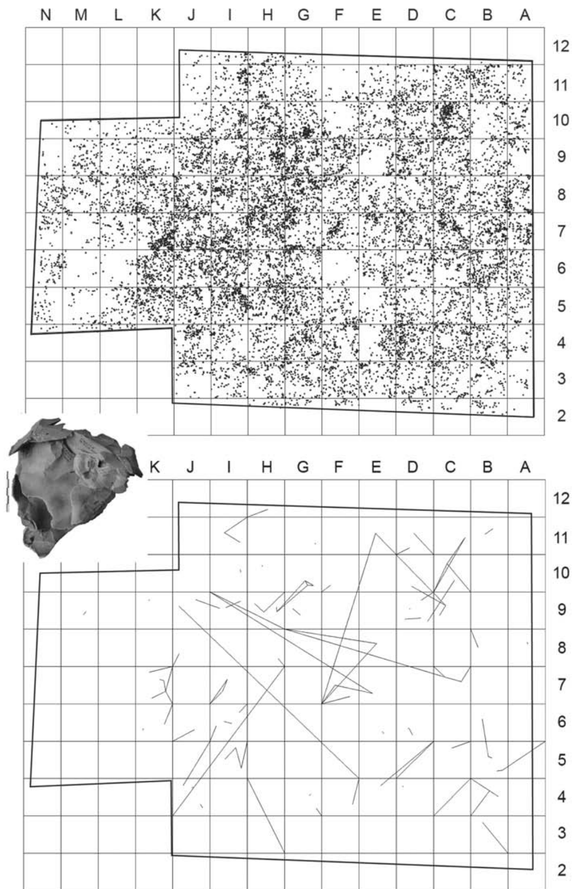
Fig. 11 : Répartition spatiale des artefacts, et des raccords et des remontages effectués.
