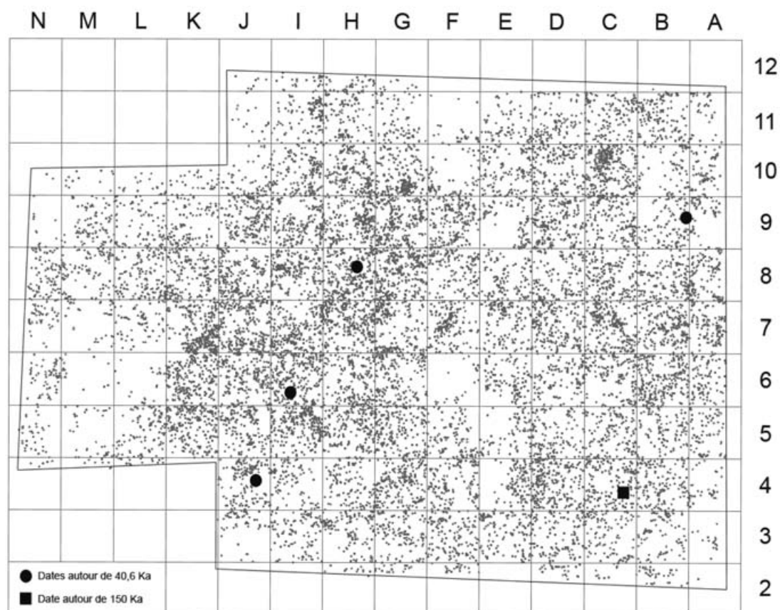
Fig. 12 : Localisation des silex chauffés sur le site d'atelier.
