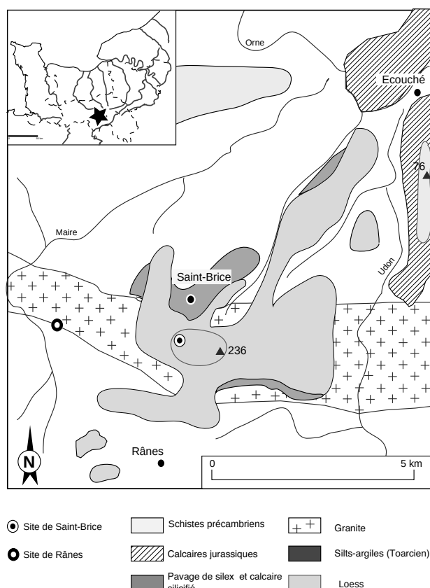
Fig. 3 : Croquis morphologique du site. Fig. 3: Morphological diagram.
