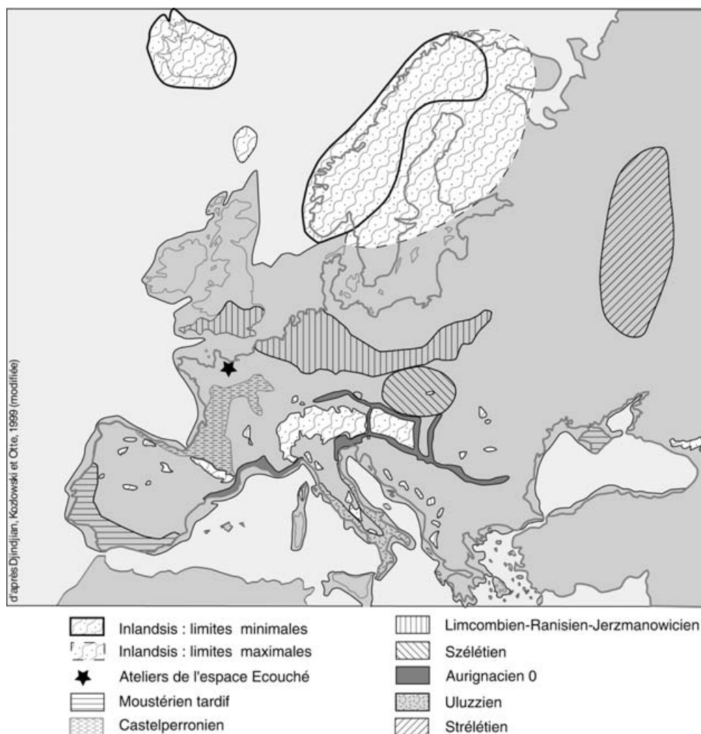
Fig. 14 : Extension des groupes culturels de la transition Paléolithique moyen / Paléolithique supérieur en Europe.
