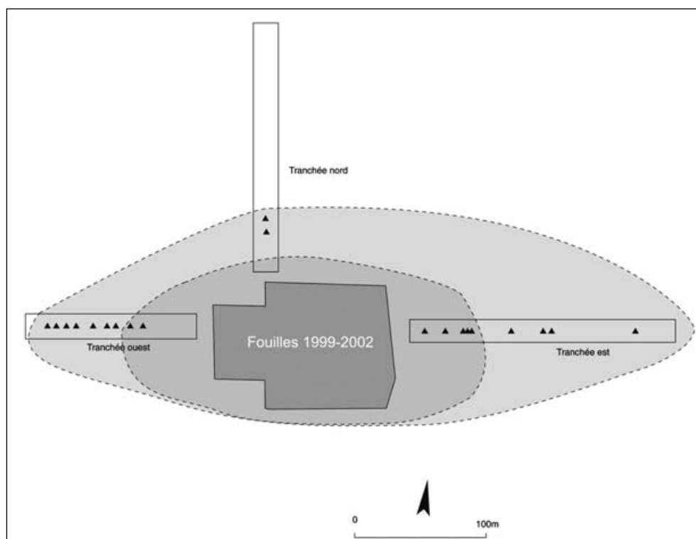
Fig. 2 : Morphologie de la nappe de vestiges du site P6 de Saint-Brice-sous-Rânes. Fig. 2: Morphology of the P6 Saint-Brice-sous-Rânes site artifact layer.
