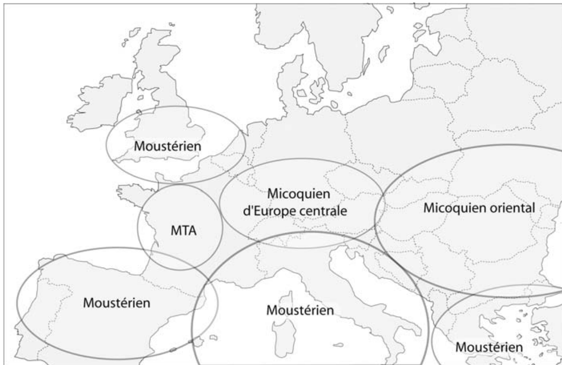
Fig. 13 : Traditions culturelles de la fin du Paléolithique moyen, en Europe (d'après Richter, 2006).
