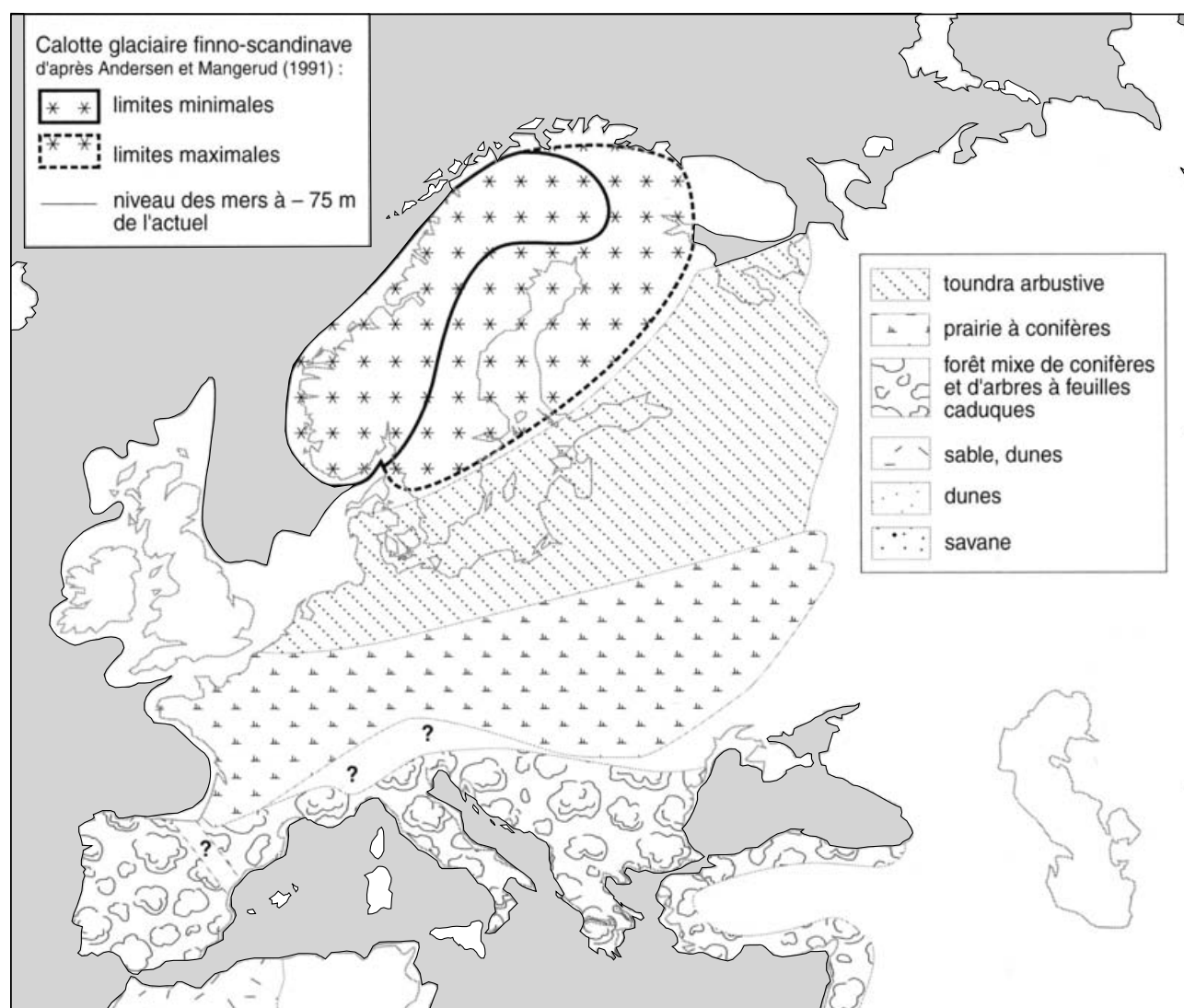
Fig. 15: Carte de la végétation en Europe pendant l'interpléniglaciaire (d'après Van Andel & Tzedakis, 1996). Fig. 15: Map of the vegetation in Europe during the interpleniglacial (from Van Andel & Tzedakis, 1996).
