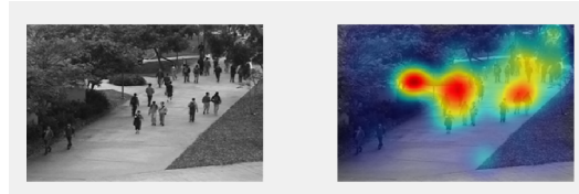
FIGURE 2 – Carte de saillance, les piétons en mouvement sont bien captés par l'approche utilisée.
