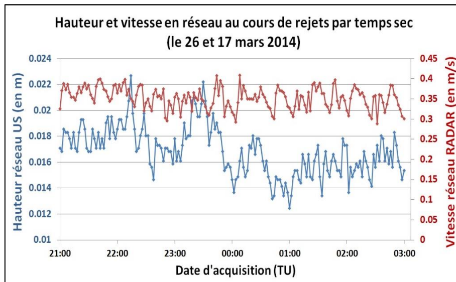
Figure 9. Hauteur d'eau et vitesse d'écoulement par temps sec avec l'ancienne station.
