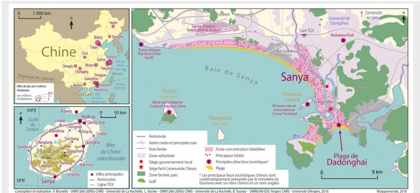
Figure 1. La plage de Dadonghai à Sanya dans le sud de l'île de Hainan (Chine). Le quartier/station de Dadonghai est l'endroit le plus populaire de la ville touristique de Sanya pour venir à la plage. Sanya est la deuxième ville (600 000 habitants) de la province de Hainan qui abrite une population d'un peu plus de 8 millions d'habitants dans une île de 33 000 km 2 à la superficie comparable à celle de Taiwan ou de la Belgique. Sanya est aussi la principale destination touristique de cette île qui reçoit chaque année plus de 40 millions de touristes du continent (moins de 1% de la fréquentation est composée de touristes étrangers, essentiellement des Russes et des Chinois de la diaspora).
