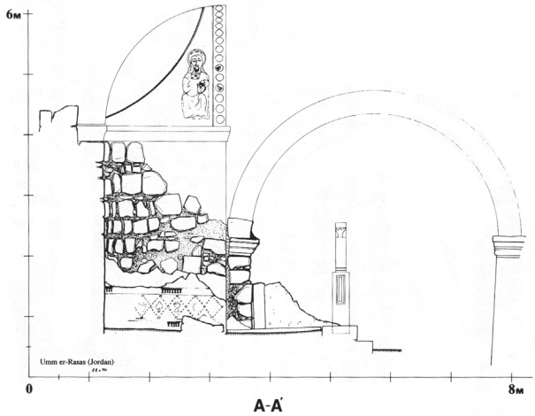
Figure 24 – Umm al-Rasas, église de Wa'il, coupe longitudinale de l'abside, restitution du décor peint de la calotte absidale couvrant la maçonnerie et relevé de l'enduit pariétal sur le mur sud du sanctuaire. [Dessin E. Alliata, T. Walisewski, dans Piccirillo 1993b, fig. 9 p. 316]
