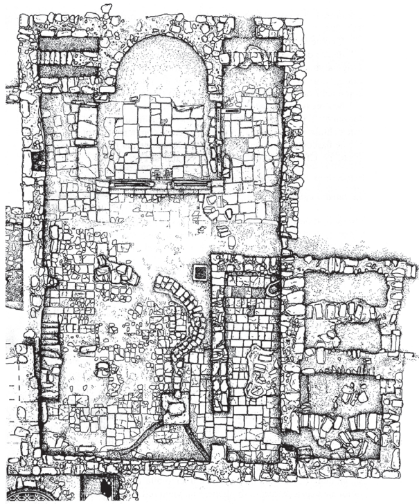
Figure 23 – Umm al-Rasas, église de la Tabula Ansata. Le relevé pierre à pierre prend en compte les irrégularités de la maçonnerie et les liaisons entre les murs. [Relevé M. Forgia, S. Deruvo, dans Piccirillo 2003, fig. 2a, p. 291]
