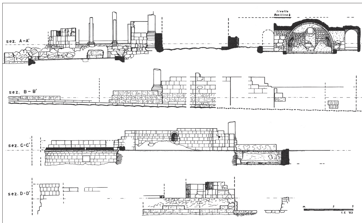
Figure 7 – Relevés d’élévations et coupe des églises de la Vierge et du prophète Élie de Madaba. [Levé et dessin E. Alliaia 1982, dans Piccirillo 1989b, p. 63]
