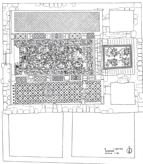
Figure 8 – Plan de l'église du diacre Thomas à 'Ayoun Mousa. Un relevé pierre à pierre partiel des maçonneries est effectué. [Dessin E. Alliaa, S. Ognibene 1986-1988, dans Piccirillo 1989b, p. 217]
