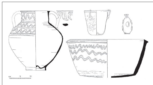
Figure 11 – Planches présentant de la céramique provenant d'Umm al-Rasas. [Dessins E. Alliata, dans Piccirillo 1989b, p. 346]
