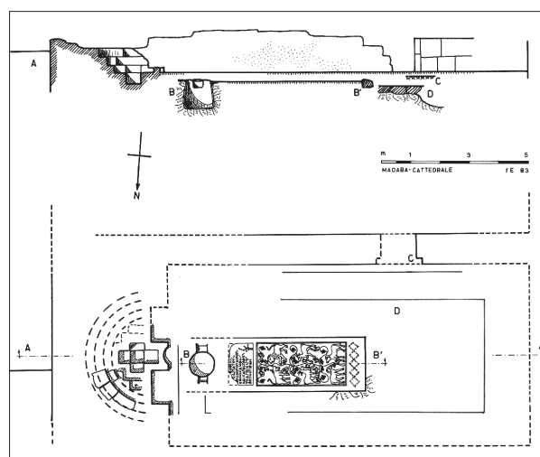
Figure 5 – Plan et coupe du baptistère fouillé en 1979-1981. Outre l'échelle, l'orientation et les traits de coupes, le dessin utilise des trames pour différencier les matériaux (hachures, pointillés, lignes tiretées). [Levé et dessin E. Alliata 1983, dans Piccirillo 1989b, p. 32]
