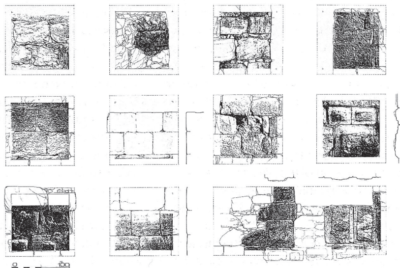
Figure 28 – Analyse des différents types d'appareils de la basilique du Nébo. [Piccirillo, Alliata 1998, fig. 13, p. 587]
