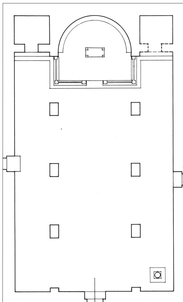
Figure 2 – Plan de Saint-Basile de Rihab. Dépourvu d'échelle et d'orientation, le dessin, schématisique, ne rend compte que des grandes masses architecturales. [Dessin C. Calano 1977-1978, dans Piccirillo 1981b, pl. 54]
