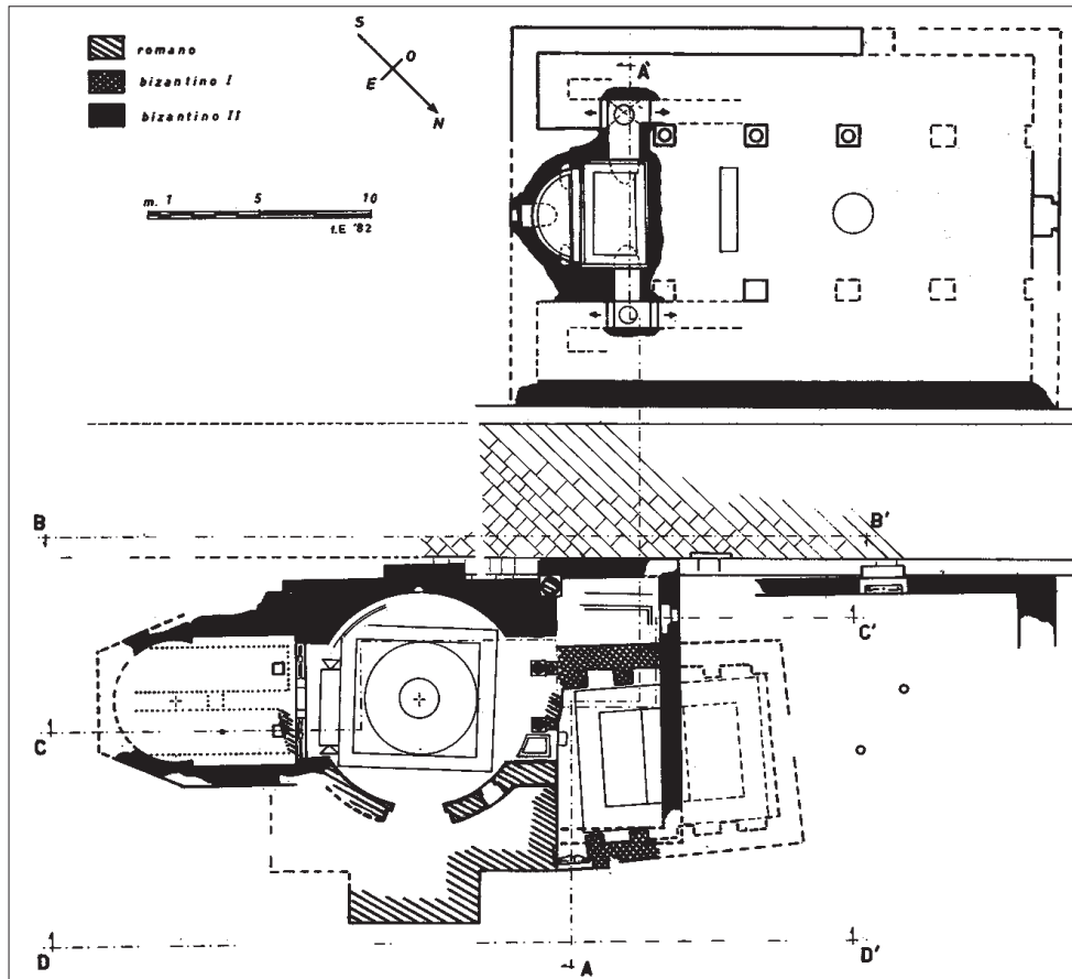
Figure 6 – Plan des églises de la Vierge et du prophète Élie de part et d’autre de la voie romaine. Les trames sont utilisées pour différencier les phases chronologiques de l’édifice. [Levé et dessin E. Alliaia 1982, dans Piccirillo 1989b, p. 62]
