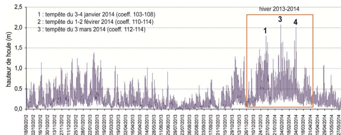
Figure D – Enregistrement de hauteur de houle à partir du capteur de pression installé dans la zone intertidale au droit du profil B, montrant les 3 épisodes tempétueux majeurs de l'hiver 2013-2014 (Fichaut et al., 2015).
