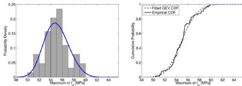
Fig. 5 – Densité de probabilité et probabilité cumulée déterminées avec la méthode du maximum de vraisemblance à partir des valeurs extrêmes de l'indicateur de fatigue mésoscopique de Dang Van pour un chargement de traction alternée symétrique
