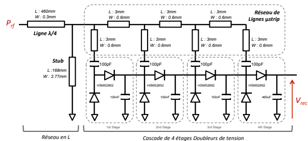
Figure 1. Architecture d'un convertisseur RF/DC
