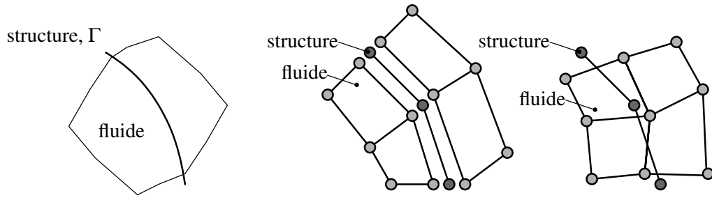
a) Fluide séparé en 2 parties par une structure b) Maillage compatible c) Maillage incompatible
