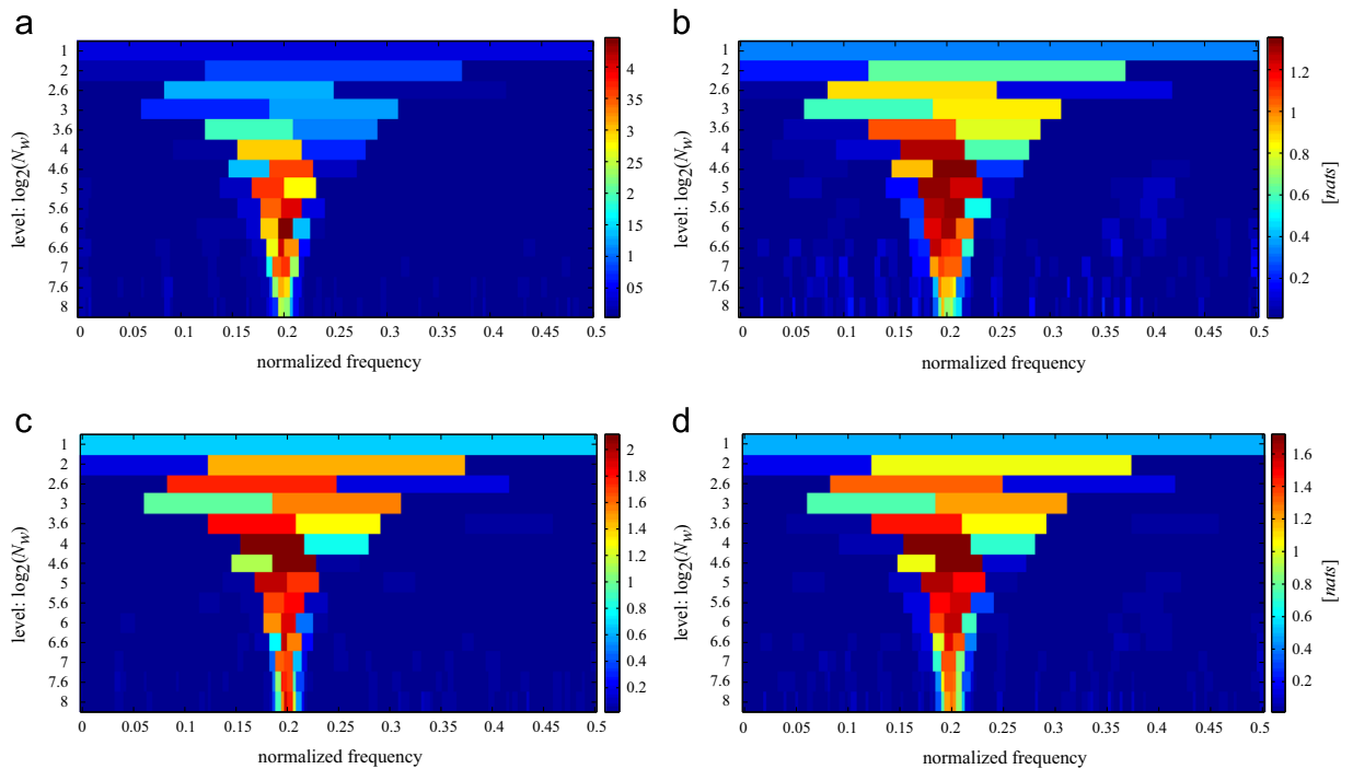
Fig. 11. (a) Kurtogram, (b) SE infogram \Delta I_e(f; \Delta f) , (c) SES infogram \Delta I_E(f; \Delta f) , (d) average infogram \Delta I_{1/2}(f; \Delta f) . Case with N = 1000 .
