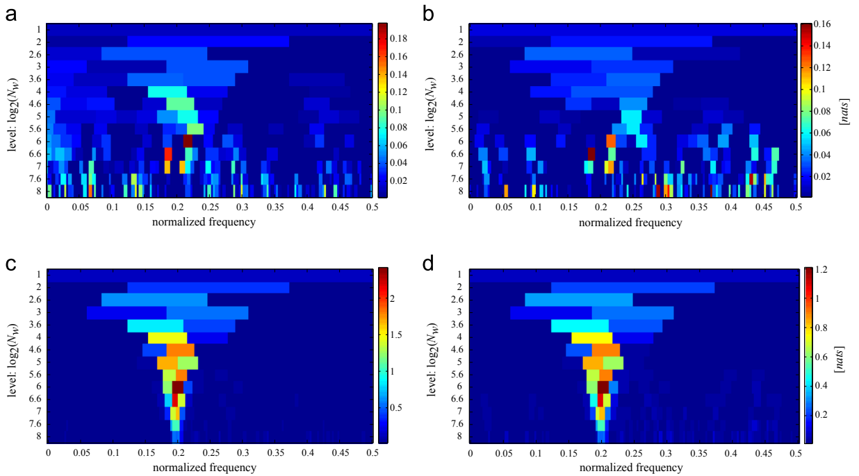
Fig. 10. (a) Kurtogram, (b) SE infogram \Delta I_e(f; \Delta f) , (c) SES infogram \Delta I_E(f; \Delta f) , (d) average infogram \Delta I_{1/2}(f; \Delta f) . Case with N = 200 .
