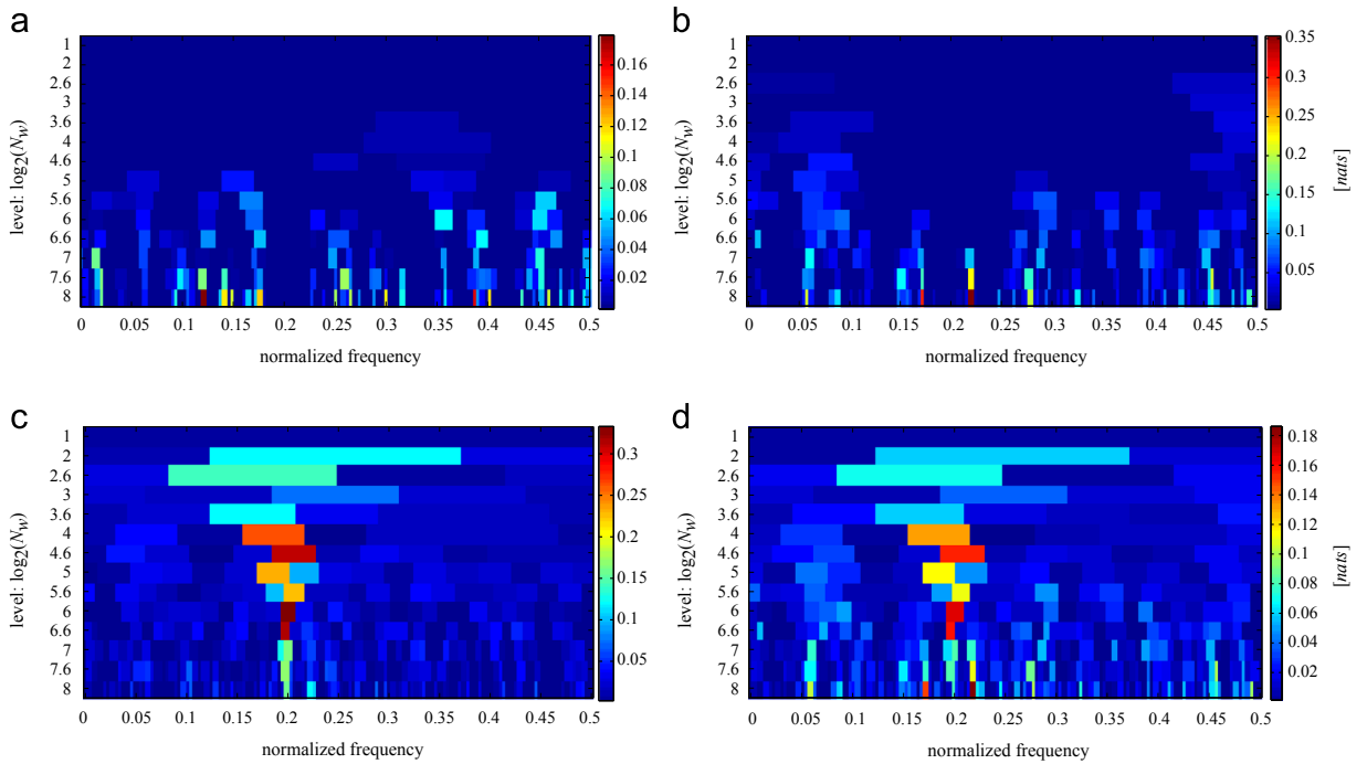
Fig. 9. (a) Kurtogram, (b) SE infogram \Delta I_e(f; \Delta f) , (c) SES infogram \Delta I_e(f; \Delta f) , (d) average infogram \Delta I_{1/2}(f; \Delta f) . Case with N = 50 .
