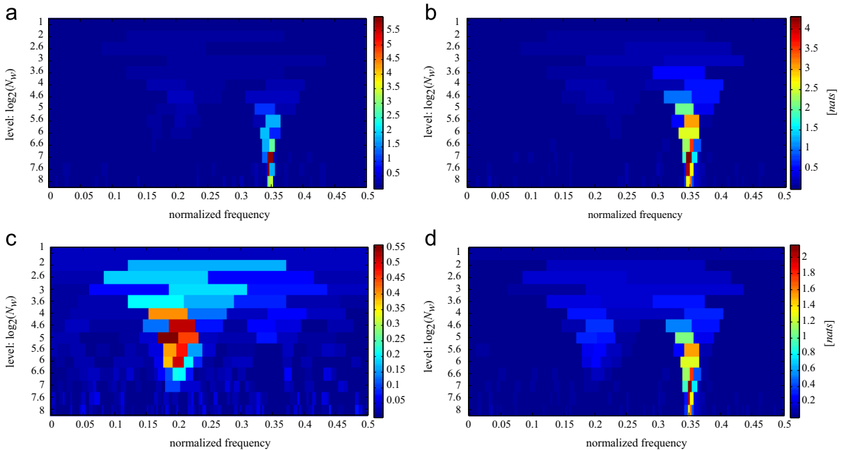
Fig. 7. (a) Kurtogram, (b) SE infogram \Delta I_e(f; \Delta f) , (c) SES infogram \Delta I_E(f; \Delta f) , (d) average infogram \Delta I_{1/2}(f; \Delta f) of the signal in Fig. 6.
