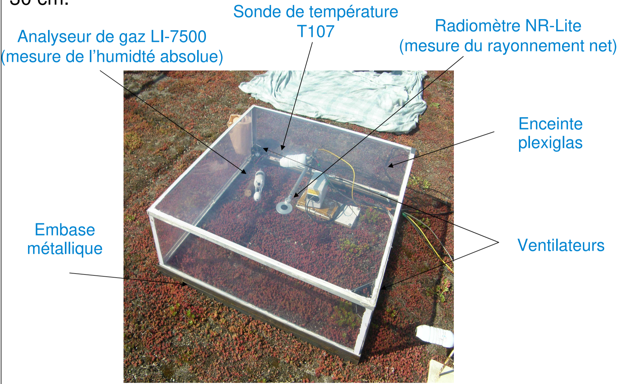
Figure 1 : Photographie de la chambre à évapotranspiration du Cerema et de ses composants.
