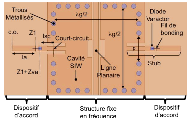
Figure 1. Illustration du résonateur coupe-bande SIW.
