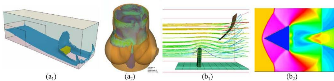
Figure 4 – illustrations de calculs réalisés : pour le solveur ICFD : (a1) rupture de barrage, (a2) valve de cœur ; pour le solveur CESE : (b1) structure souple dans un fluide subsonique, (b2) visualisation d'ondes de choc
