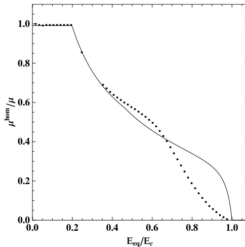
FIGURE 2 – Comparaison du comportement homogénéisé pour le module de cisaillement \mu^{\text{hom}} (normée par le module de cisaillement des éléments volumiques \mu ) en fonction du chargement imposé : résultat numérique par MEF (pointillés) et prédiction du modèle proposé (courbe continue).
