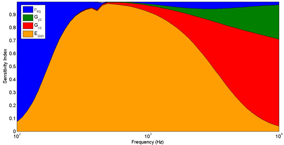
Figure 1 Indices de sensibilité des paramètres de la plaque sandwich
