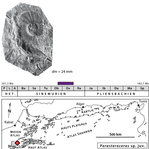
Fig. 88: Parasteroceras sp., dm = 24 mm, coupe de Taguendouf (près de Ouauoiserth), niv. 516, Haut Atlas de Béni Mellal, Maroc [El Hariri et al. , 1996, pl. 67, fig. 21, modifié].
