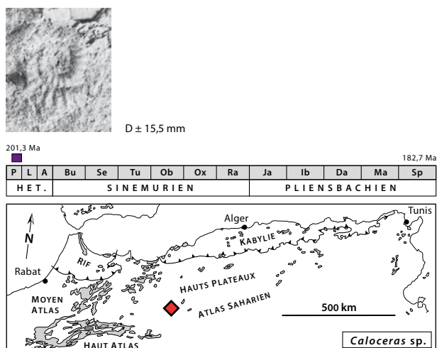
Fig. 48: Caloceras sp., D \approx 15,5 mm, Coupe du Djebel Chemarikh, Mont des Ksour, Algérie [Elmi et al. , 1998, p. 169, fig. 11(e) modifié].
