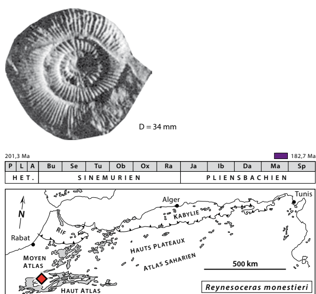
Fig. 182: Reynesoceras monestieri (Dubar & Mouterde, 1978), D = 34 mm, Cherket, Haut Atlas du Tadla, Maroc [Dubar & Mouterde, 1978, pl. 3, fig. 6, modifié].
