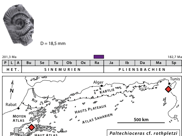
Fig. 117: Paltechioceras cf. rothpletzi (Böse, 1894), D = 18,5 mm, Kadoussa, Haut Atlas, Maroc [Guex et al. , 2008, pl. 17, fig. 8, modifié].
