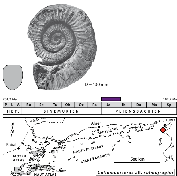
Fig. 136: Callomonicer aff. salmojraghii (Parona, 1894), D = 130 mm, Djebel Oust, probablement niveau 7, Dorsale tunisienne, Tunisie [Rakús & Guex, 2002, pl. 18, fig. 1, text-fig. 81a, modifié].
