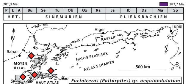
Fig. 203: Fuciniceras (Paltarpites) gr. aequiondulatum (Bettoni, 1900), à gauche dm = 29 mm, au centre D = 27 mm, Toughza, Béni Mellal [El Hariri et al. , 1996, pl. 71, fig. 6, modifié]; à droite, D = 33 mm, Djebel Bou Rharraf [Meister et al. , 2011, p. 117.e42, fig. 23(4), modifié].
