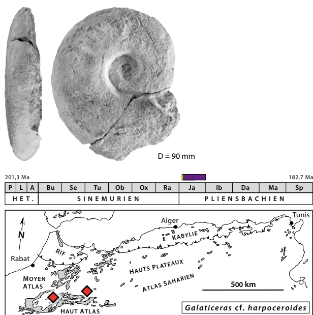
Fig. 20: Galaticeras cf. harpoceroides (Gemmellaro, 1884), D = 90 mm, Bou Rharraf, Haut Atlas oriental, Maroc [Meister et al. , 2011, p. 117.e14, fig. 9(3), modifié].
