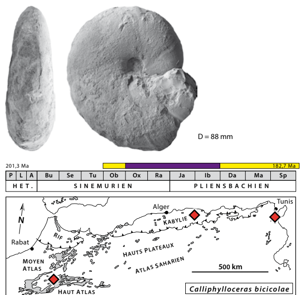
Fig. 4: Calliphyloceras bicolae (Meneghini, 1874), D = 88 mm, Grande Kabylie, Algérie [Dommergues et al. , 2008, p. 547, fig. 3(B, C), modifié].
