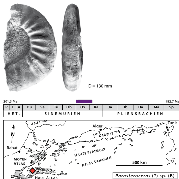
Fig. 90: Parasteroceras (?) sp. (B), D = 130 mm, Foug Tillicht, niv 4.1, Haut Atlas, secteur de Midelt, Maroc [Wilmsen et al. , 2002, pl. 2, fig. 2, modifié].
