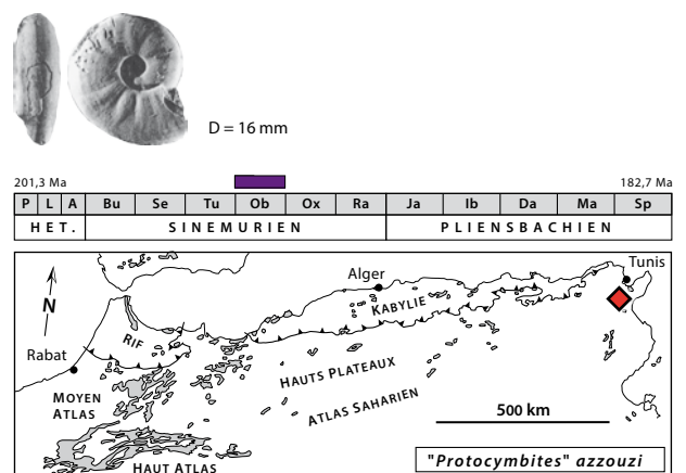
Fig. 125: « Protocymbites » azzouzi Rakús & Guex, 2002, holotype, D = 16 mm, Djebel Oust, niveau 4-5, Dorsale Tunisienne, Tunisie [Rakús & Guex, 2002, pl. 12, fig. 4, 5, modifié].
