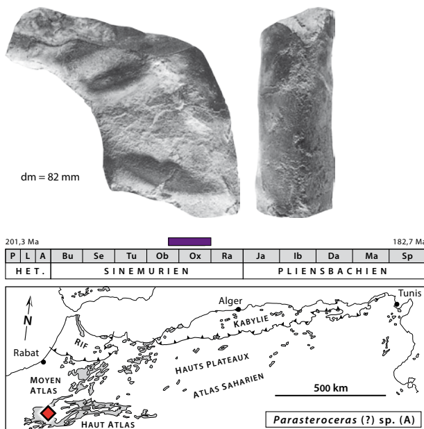
Fig. 89: Parasteroceras (?) sp. (A), dm = 82 mm, coupe de Taguendouf (près de Ouauoiserth), niv. 517, Haut Atlas, secteur de Béni Mellal, Maroc [El Hariri et al. , 1996, pl. 67, fig. 19, 20, modifié].
