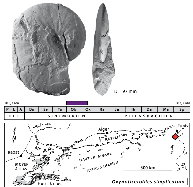
Fig. 106: Oxynoticeroides simplicatum Dommergues, Fauré & Peybernes, 1986, holotype, D = 97 mm, carrières au sud-est du Djebel Oust, niveau (b), Dorsale tunisienne, Tunisie [nouvelles photographies correspondant au spécimen préalablement illustré par Dommergues et al. (1986, pl. 1, fig. 7)].
