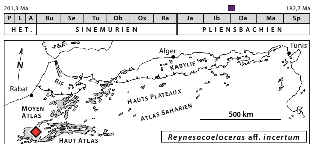
Fig. 167: Reynesocoeloceras aff. incertum (Fucini, 1905), D = 43 mm, coupe de Taguendouf, niveau 1058, Ouaouizerth, Haut Atlas secteur de Béni Mellal, Maroc [El Hariri et al. , 1996, pl. 70, fig. 5, 6, modifié].
