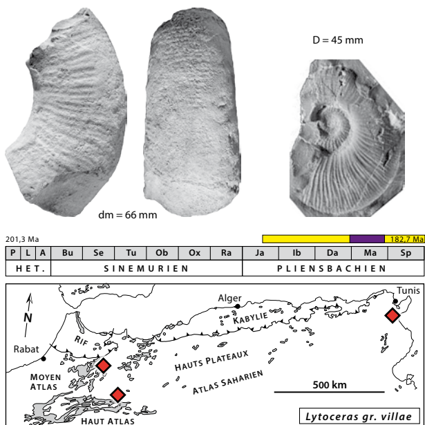
Fig. 37: Lytoceras gr. villae Meneghini, 1874, à gauche dm = 66 mm, Haut Atlas, Bou Rharraf, Maroc [Meister et al. , 2011, p. 117.e12, fig. 8(4), modifié], à droite D = 45 mm, Moyen Atlas septentrional, Merhraoua, Maroc [Morard, 2004, pl. 1, fig. 8, modifié].
