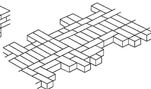
d) M 140, Warka/Uruk, Eanna, niveau IV (d'après Heinrich, 1934, fig. 20)
