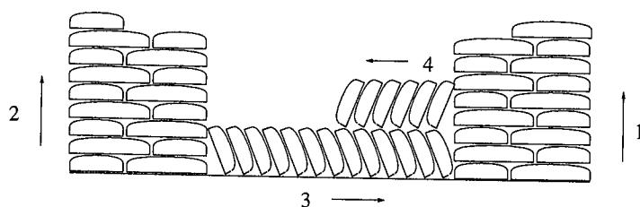
Fig. 69. - Mode d'élaboration d'un mur en arête de poisson (d'après Delougaz, 1933, fig. 23, p. 24).
