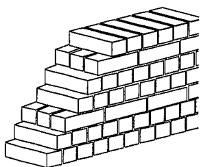
c) M 165, Asmar/Ešnunna Temple d'Abu, Archaic Shrine III (d'après Delougaz et Lloyd, 1942, fig. 127, p. 169 et fig. 128, p. 170)
