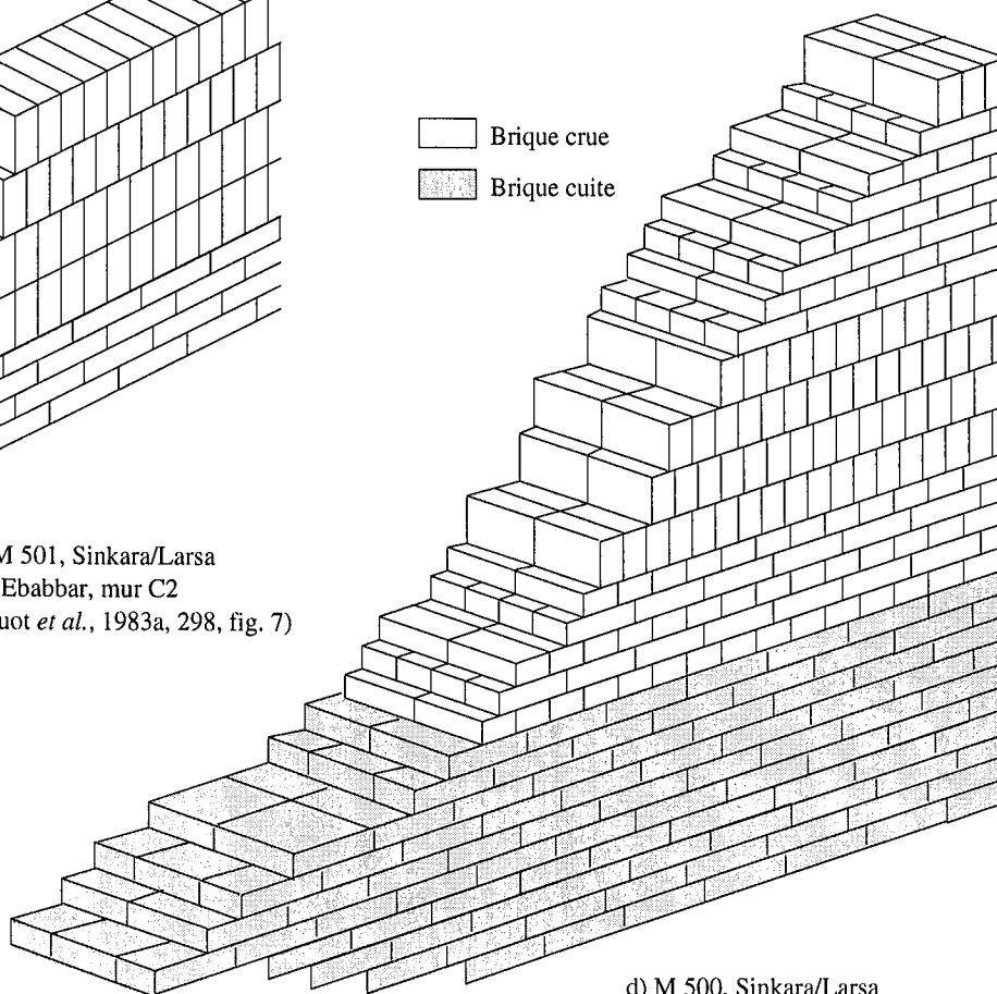
d) M 500, Sinkara/Larsa Ebabbar, pièce 23 (d'après Huot et al. , 1987b, 180, fig. 33)
