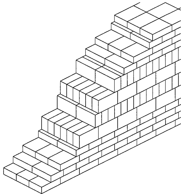
c) M 316, Muqqayar/Ur Ziggurat d'Ur Nammu, cœur de briques crues (d'après Woolley, 1939, fig. 10, p. 113)
