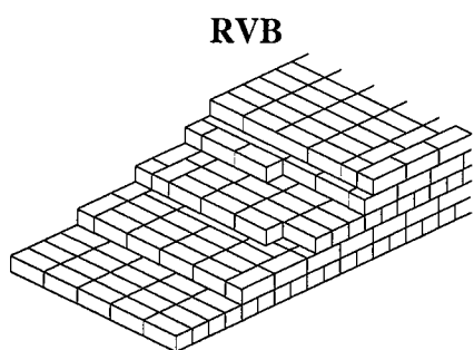
Fig. 43. - Riemchenverband .
