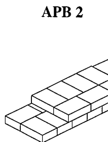
Fig. 46. - Appareil alternant rangs de panneresses et rangs de boutisses sur une même assise.
