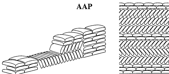
Fig. 44. - Appareils en arête de poisson.
