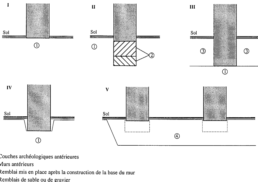
Fig. 34. – Différents types de fondations (d'après Gasche et Birschmeier, 1981, fig. 4, p. 16).
