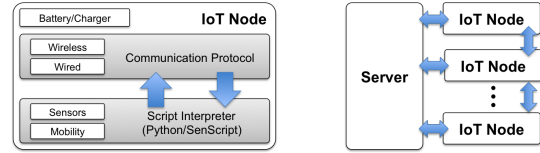
Fig. 4. The IoT node.
