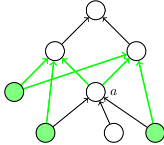
FIGURE 3. Agents permettant de calculer \mu(a) : voisins de a dans chacun de ses hôtes
