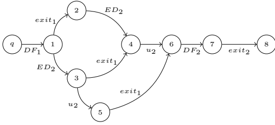
Fig. 8 Trim(NIS(S_2, q))
