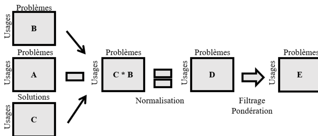
Figure 4 – Flux de données pour l'algorithme DSM-Value-Bucket
