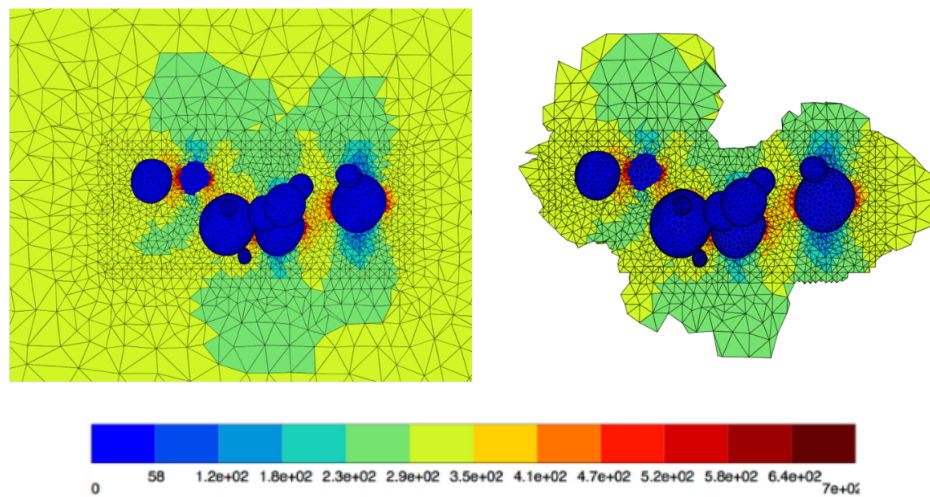
FIGURE 6 – Champ de contrainte équivalente de von Mises pour la simulation classique éléments finis (à gauche) et pour la simulation hyper-réduite (à droite)
