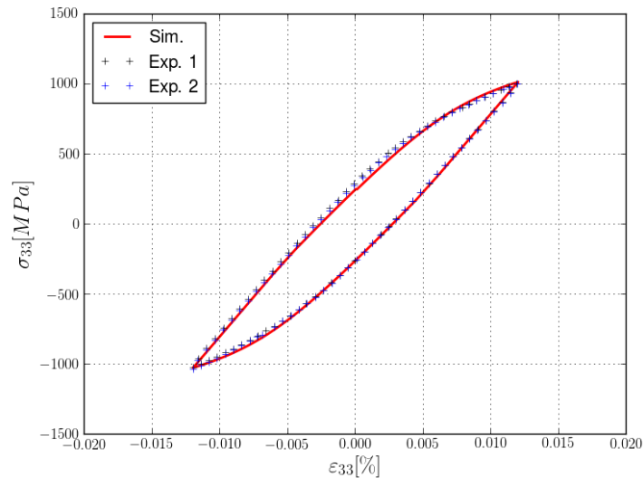
FIGURE 2 – Cycle stabilisé d'un essai d'érouissage cyclique sur TA6V- \alpha' et simulation avec le comportement élasto-visco-plastique identifié.
