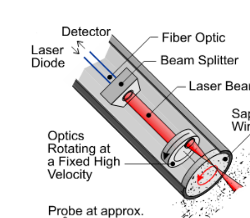
FBRM Probe
