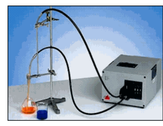
ATR Probe
