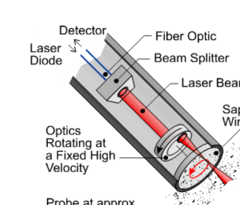
FBRM Probe
