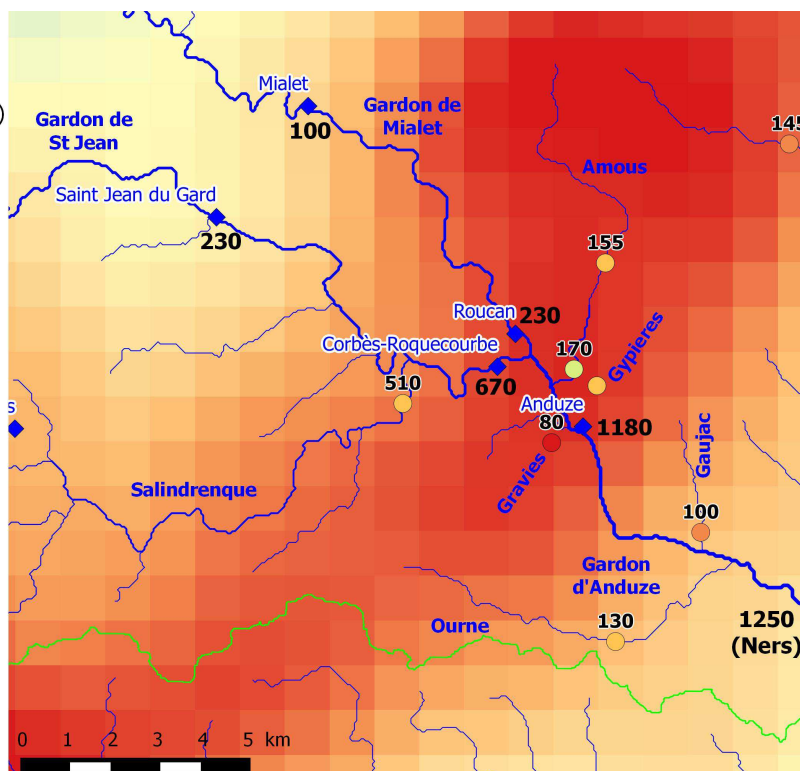
Figure 5. Estimations des débits de pointe disponibles dans le bassin aval du Gardon d'Anduze (enquête post crue et stations hydrométriques). Les débits estimés sur l'Amous correspondent à la crue du 20/9. Les cumuls de pluie présentés sont donnés à titre indicatif et concernent la période du 15/9 06:00 au 20/09 06:00.
