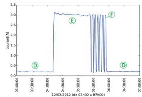
Figure 4 - Exemple de consommation d'un système de télécommunication.
