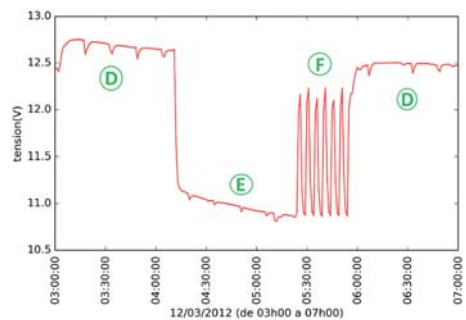
Figure 5 - Événement de surconsommation, mesure du courant de consommation et tension de batterie.
