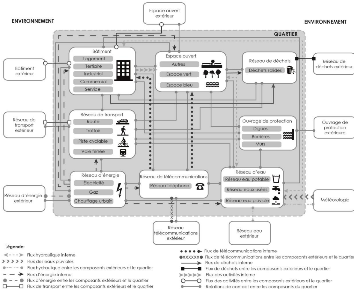
Figure 4. Bloc-diagramme Fonctionnel du système quartier (Balsells et al., 2013b)
