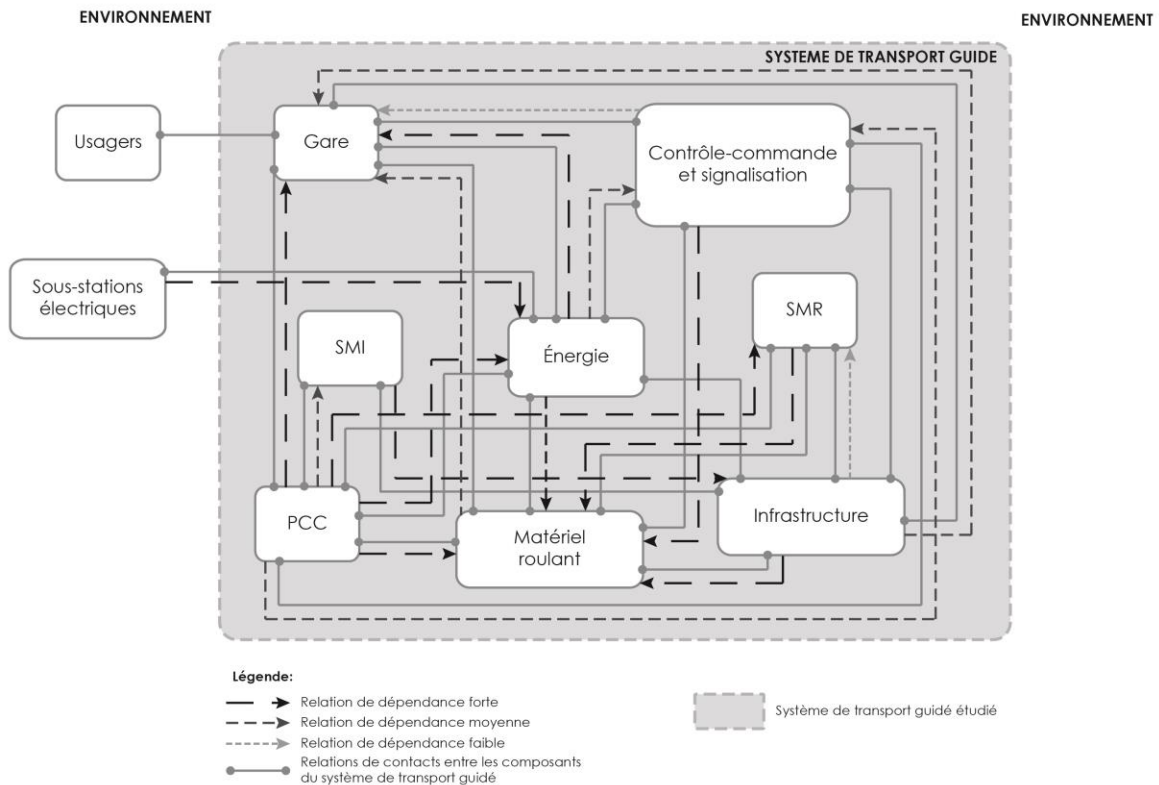
Figure 5. Bloc-diagramme Fonctionnel du système de transport guidé (auteur : Gonzva, M., 2014)
