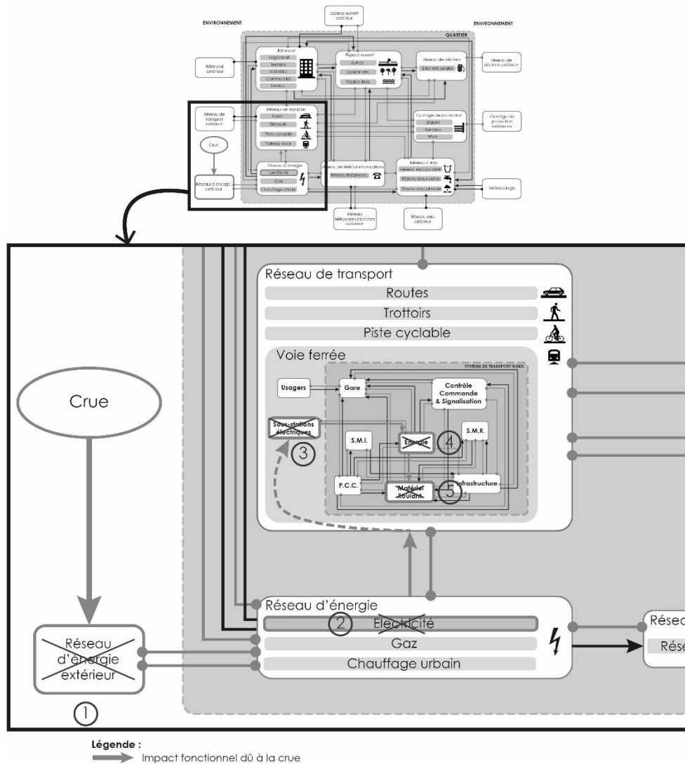
Figure 6. Imbrication des analyses fonctionnelles du quartier et du système de transport guidé (auteur : Balsells, M., Gonzva, M., 2014)
