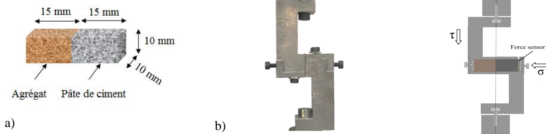
Figure 1. Dimensions des échantillons a) et dispositif expérimental pour l'essai de cisaillement direct b).
