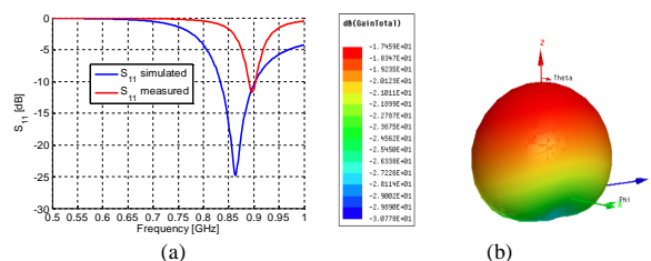
Figure 3. Coefficients de réflexion (a) et diagramme de rayonnement (b) simulés de l’antenne implantée.
