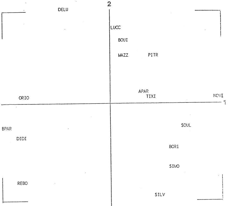
REPRESENTATION DES INDIVIDUS DANS LE PLAN 1,2
