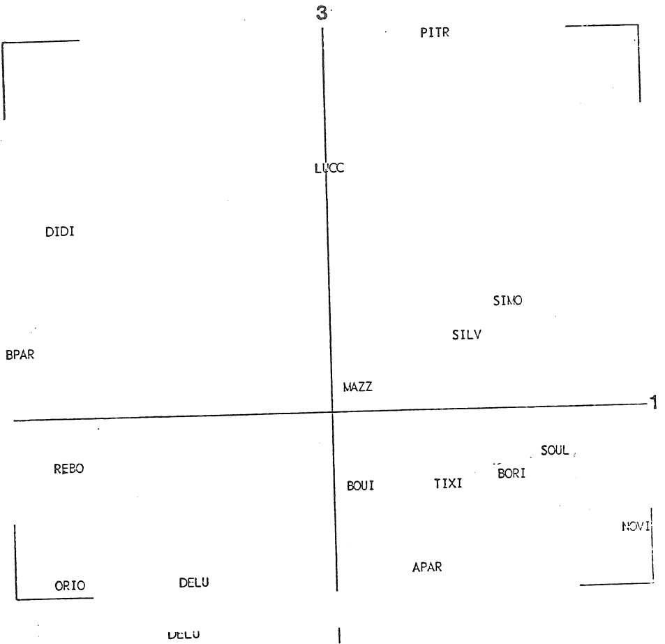
REPRESENTATION DES INDIVIDUS DANS LE PLAN 1,3
