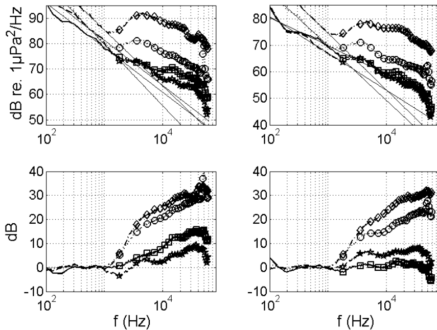
Figure 4. 95° centile (à gauche) et médiane (à droite) des spectres acoustiques en fonction du type d'habitat (losange : roche, rond : herbier, carré : coralligène, étoile : sable). En a) et b) les spectres bruts, les lignes noires sont les régressions linéaires extrapolant les niveaux sonores du bruit de l'agitation de surface, En c) et d) les spectres corrigés de la tendance linéaire afin de mettre en avant la contribution de la biophonie
