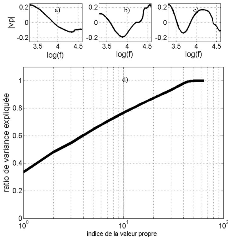
Figure 5. d) Pourcentage de variance expliquée en fonction du nombre de valeurs propres utilisées ; a),b),c) forme spectrale des trois premières composantes de l'ACP
