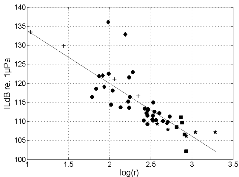
Figure 3. Niveau sonore IL large bande [2 kHz, 40 kHz] dB re.1μPa en fonction du logarithme en base 10 de la distance « r » entre la position de mesure, (N = 44) et la côte la plus proche. Losange : roche, rond : herbier, étoile : sable, carré : coralligène, croix : point fixe. Droite : meilleure régression linéaire
