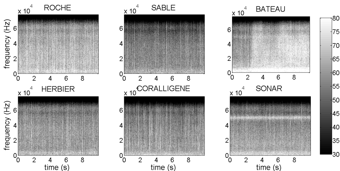
Figure 2. Spectrogrammes typiques des mesures, en haut à gauche : roche, en haut au milieu sable, en haut à droite présence d'un bateau moteur allumé, en bas à gauche herbier, en bas au milieu coralligène, en bas à droite bateau avec sondeur allumé et moteur éteint
