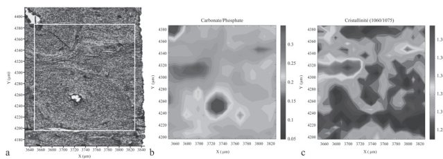
Figure 4 : (Voir planche couleur) (a) Vue optique de la zone de l'échantillon ST-Ta-8 analysée par micro-spectrométrie IR et distribution des (b) teneurs relatives en carbonates et (c) des valeurs de cristallinité dans cette même zone.
